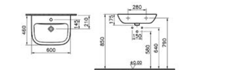
чертеж Раковина Vitra S20 5502B003-0001 (60 см.)
